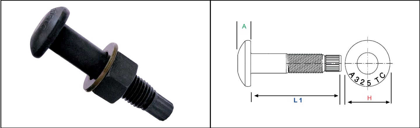
PERNO DE TORQUE CONTROLADO
