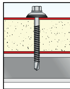
Golilla paragua F100 - CX0.
