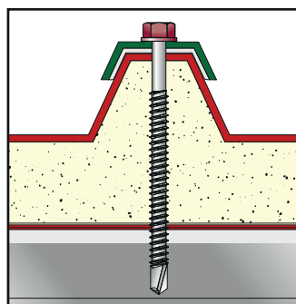
Tapón QE01 y Golilla metálica grecada AE09.
