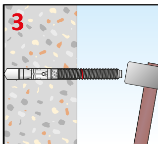
3- Golpear perno hasta la línea roja que marca la rosca.
