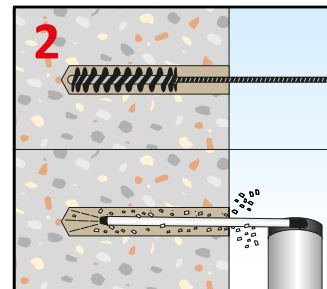
2- Limpiar zona de perforación.
