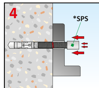
4- Coloque cilindro protector SPS, para fijar anclaje.
