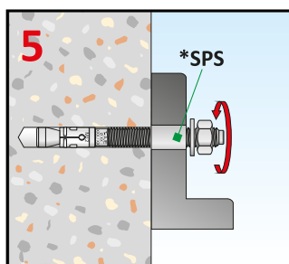
5- Coloque golilla y tuerca.
