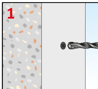
1- Hacer perforación previa.
