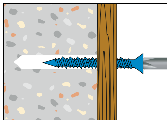
3- Coloque el soporte, inserte tornillo usando herramienta de instalación.
